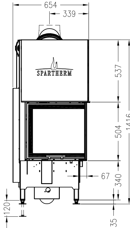
Vorderansicht M~1:20
