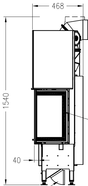
Seitenansicht M~1:20
